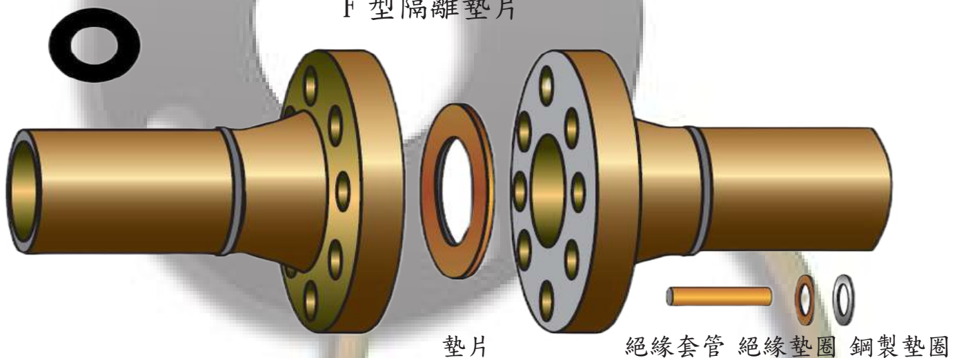
F 型隔離墊片
