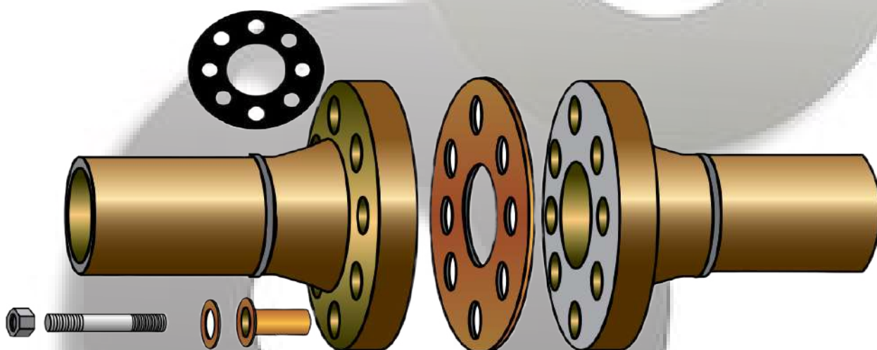
螺帽 雙頭螺柱 絕緣墊圈 一件絕緣套管和墊片
